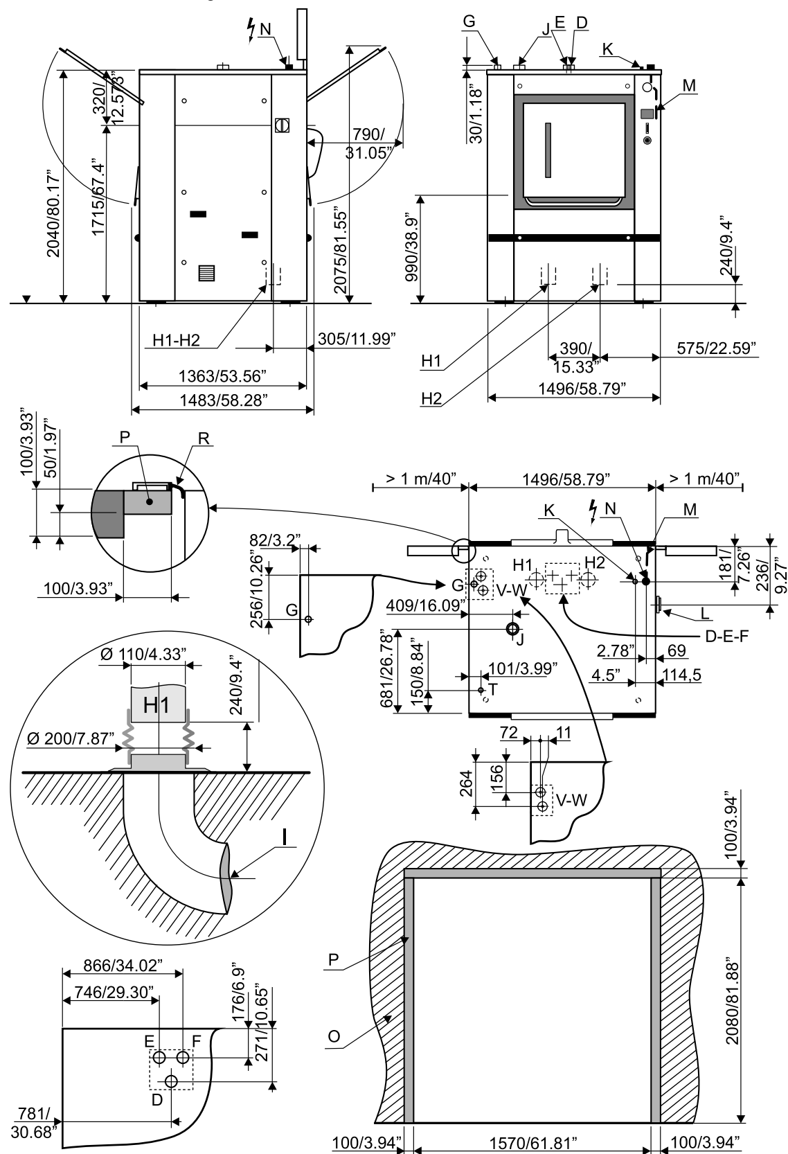
Wasmachinetype WB6 70 (Schema N° 07100157 en 07100158)
